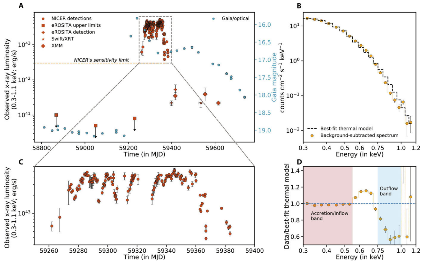
Долгосрочная эволюция ASASSN-20qс и образец рентгеновского спектра, подчеркивающий отток
