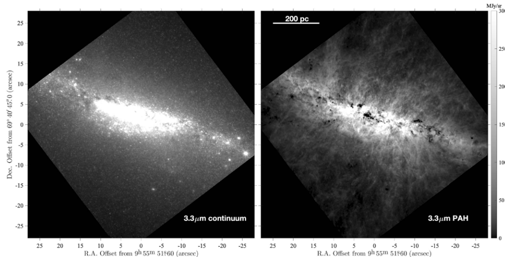
Эмиссия ПАУ, обусловленная влиянием галактического ветра
